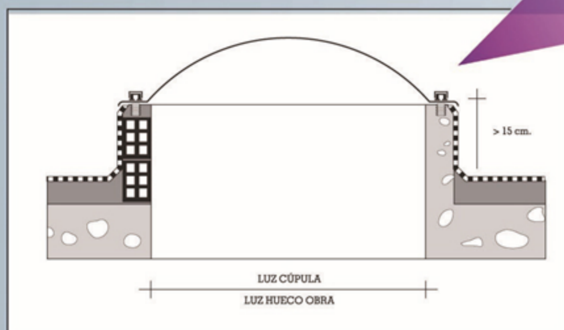
ESQUEMA INSTALACIÓN SOBRE CUBIERTAS LISAS
