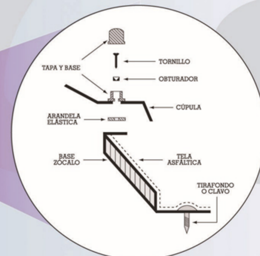
ESQUEMA DE MONTAJE DE CÚPULA SOBRE BASE-ZÓCALO
